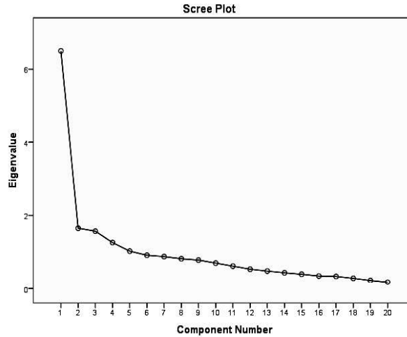
الشكل ١: مخطط الحصة لتحديد عدد العوامل
